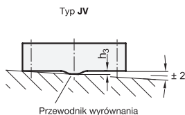
Przykład montażu
